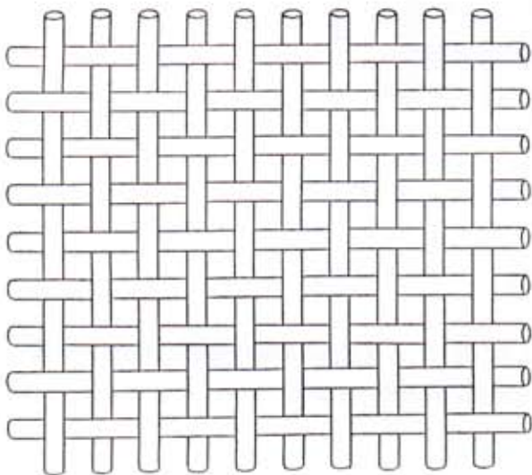
図1 平織金網
